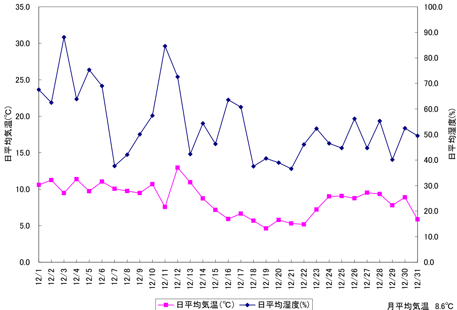
図 日平均気温と日平均湿度(東京都世田谷区用賀 2009/12/01~2009/12/31)
