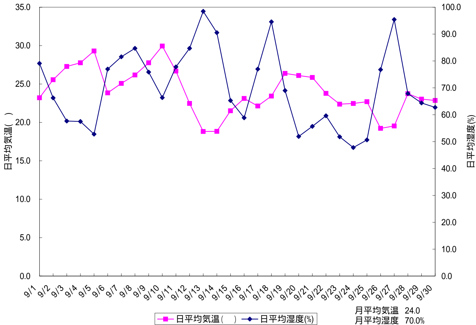
図 日平均気温と日平均湿度(東京都世田谷区用賀 2006/09/01 ~ 2006/09/30)
