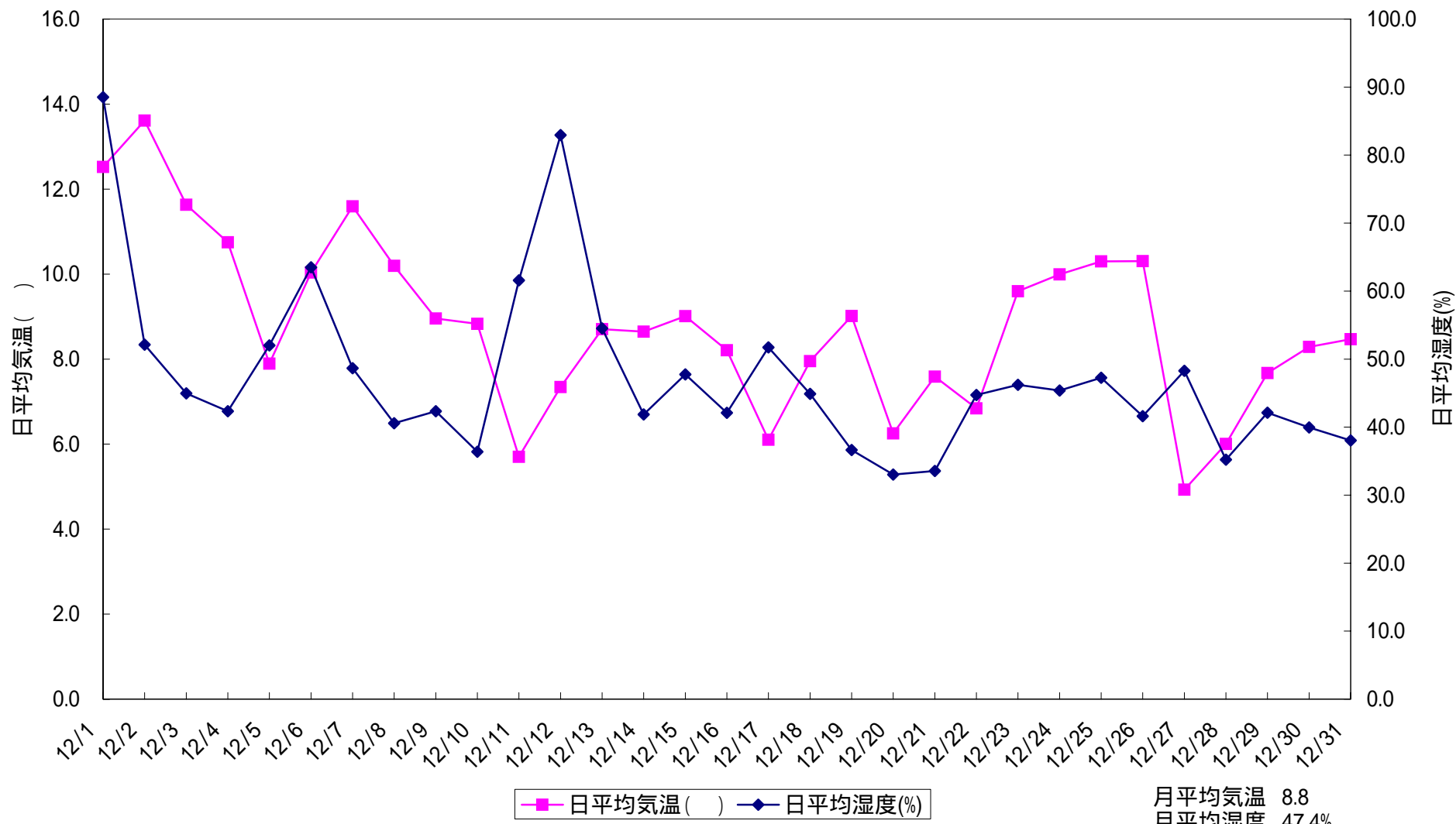
図 日平均気温と日平均湿度(東京都世田谷区用賀 2003/12)
