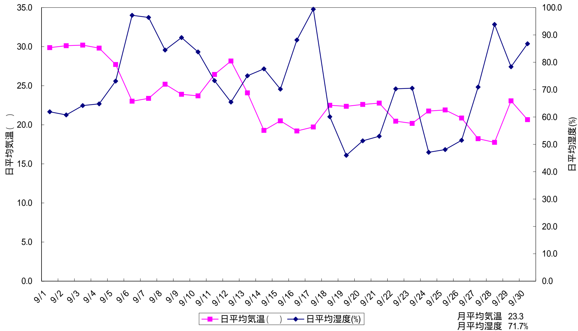
図 日平均気温と日平均湿度(2002/9 東京都世田谷区用賀)
