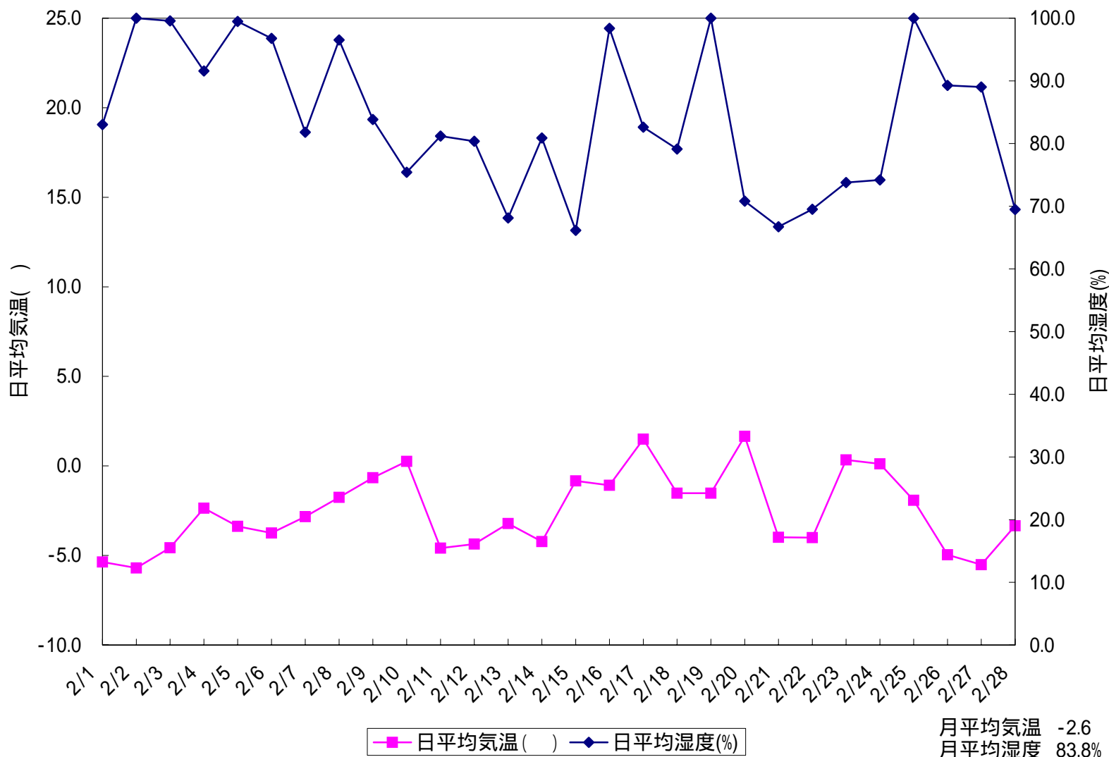
図 日平均気温と日平均湿度(群馬県川場村ヒロイド 2005/02/01 ~ 2005/02/28)
