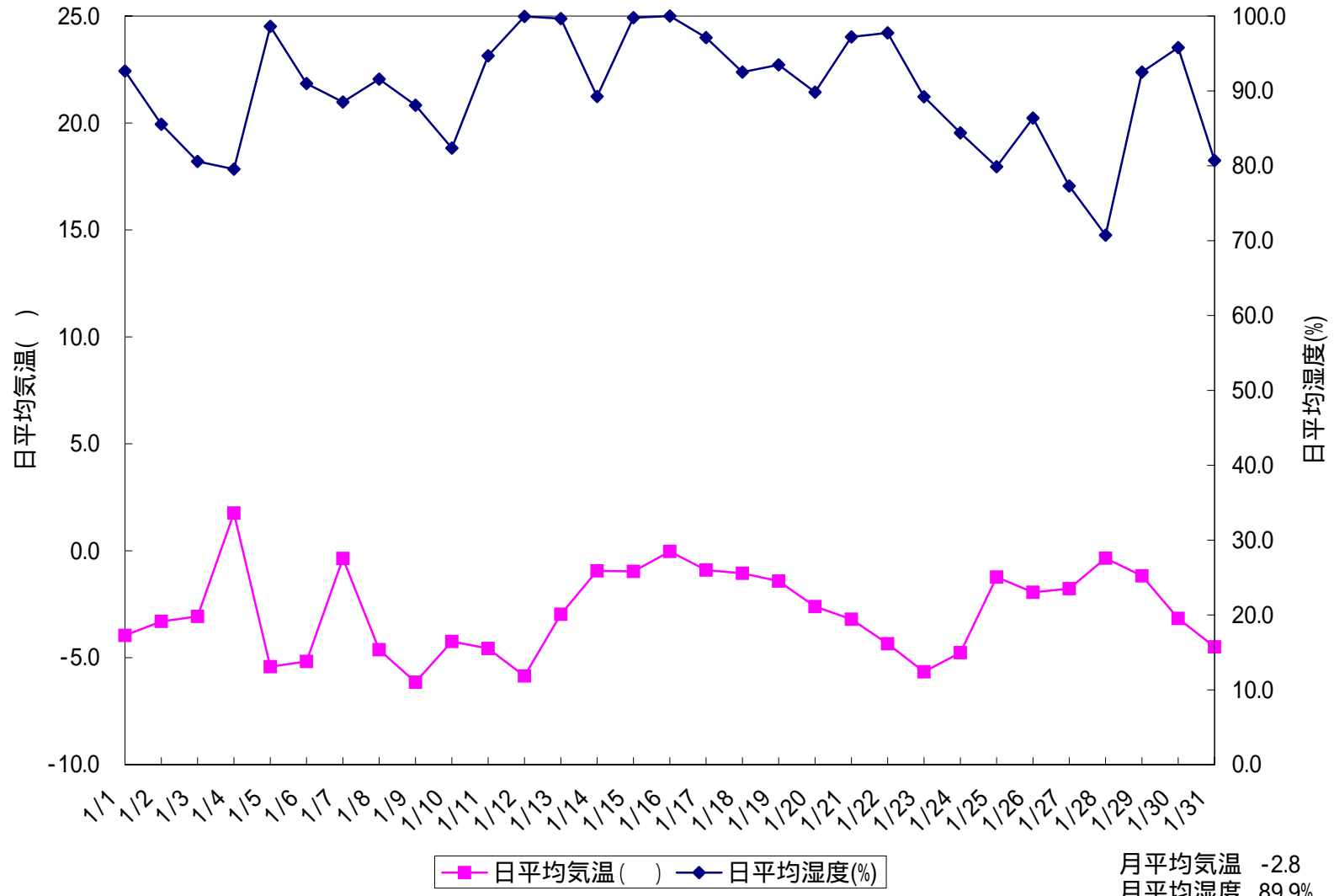
図 日平均気温と日平均湿度(群馬県川場村ヒロイド 2005/01/01 ~ 2005/01/31)
