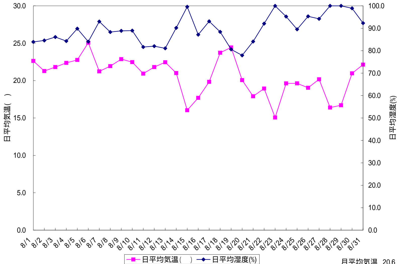
図 日平均気温と日平均湿度(群馬県川場村ヒロイド 2004/08/01 ~ 2004/08/31)
