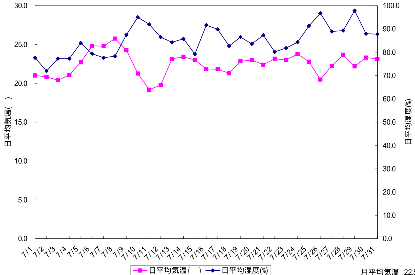
図 日平均気温と日平均湿度(群馬県川場村ヒロイド 2004/07/01 ~ 2004/07/31)
