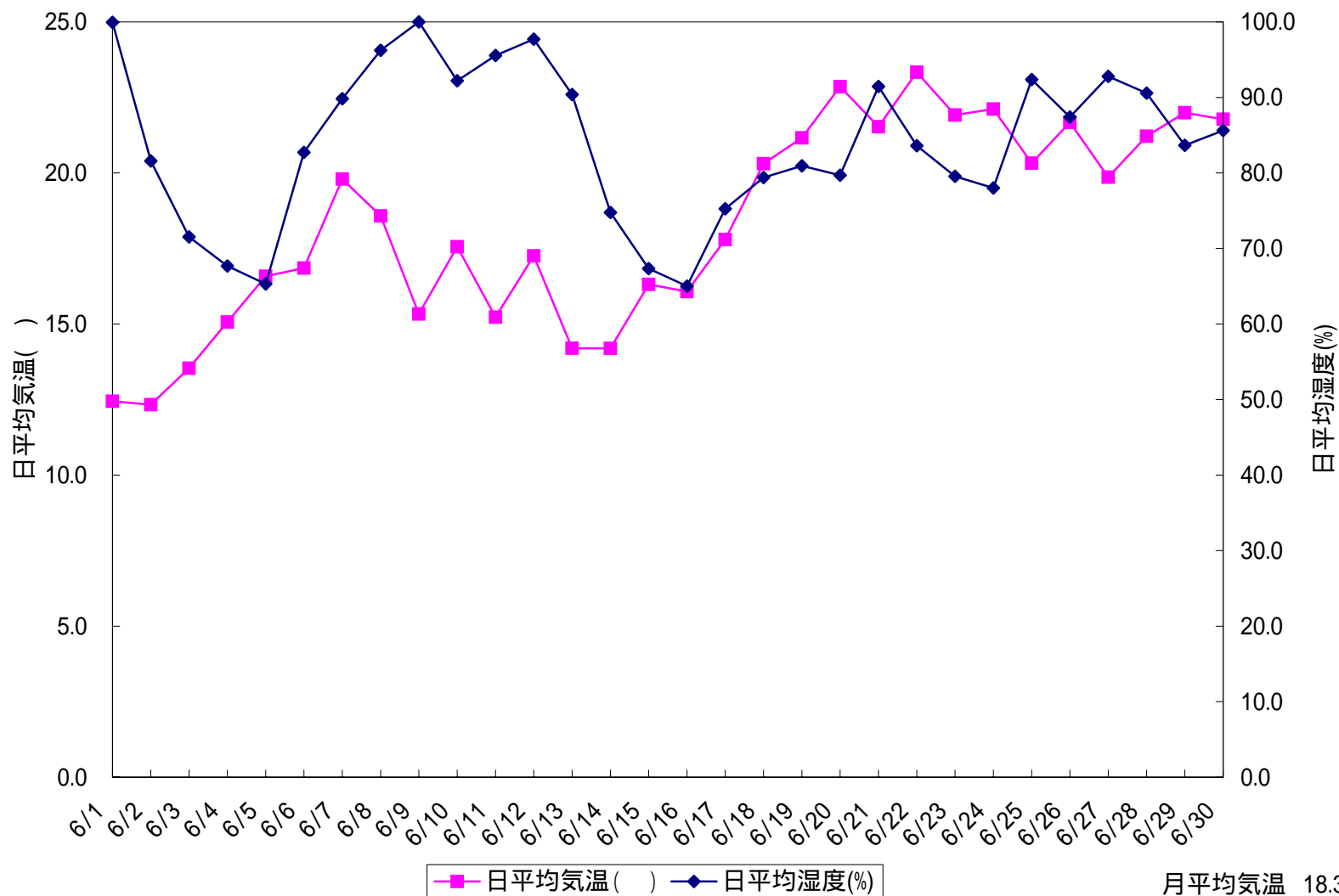
図 日平均気温と日平均湿度(群馬県川場村ヒロイド 2004/06/01 ~ 2004/06/30)
