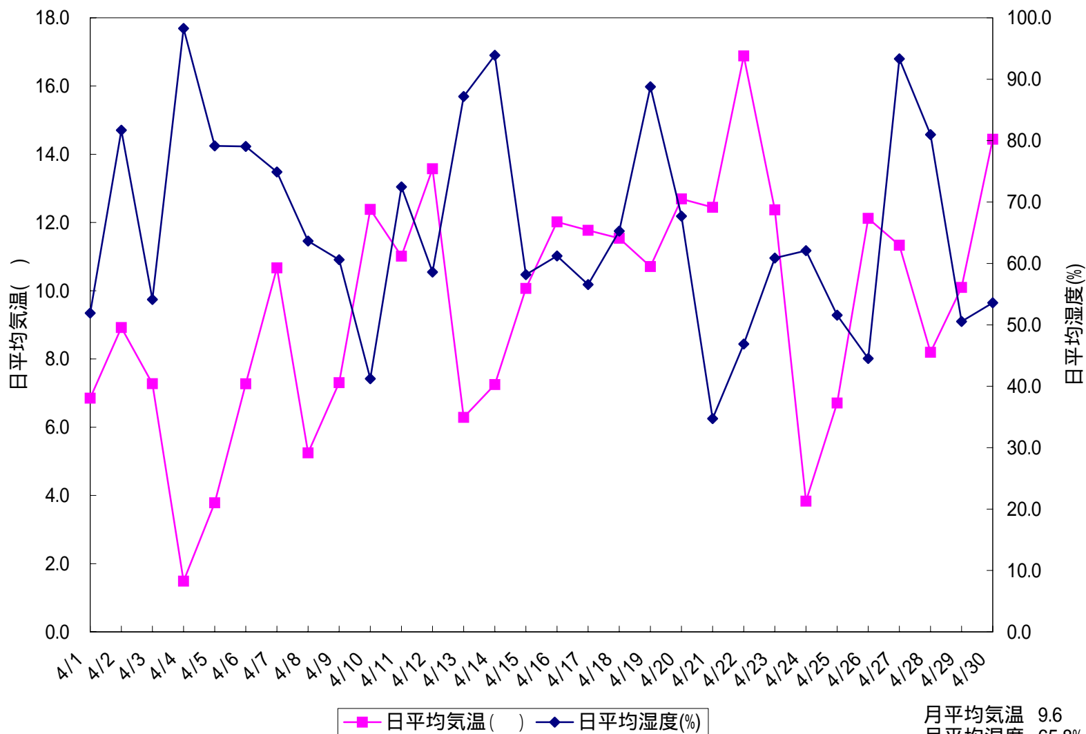
図 日平均気温と日平均湿度(群馬県川場村ヒロイド 2004/04/01 ~ 2004/04/30)
