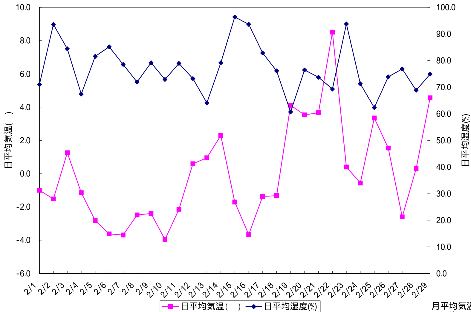
図 日平均気温と日平均湿度(群馬県川場村ヒロイド 2004/02/01 ~ 2004/02/29)
