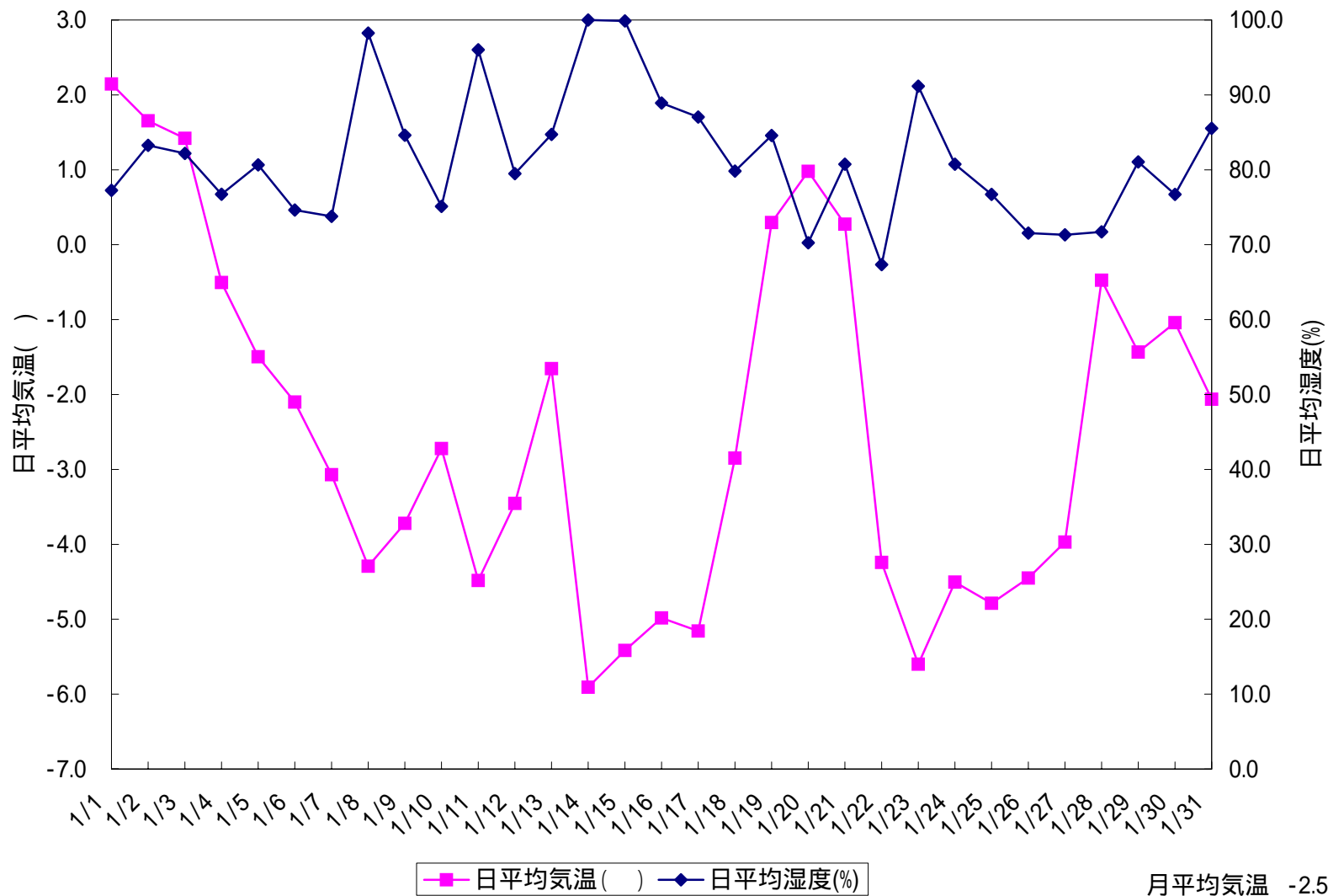
図 日平均気温と日平均湿度(群馬県川場村ヒロイド 2004/01/01 ~ 2004/01/31)
