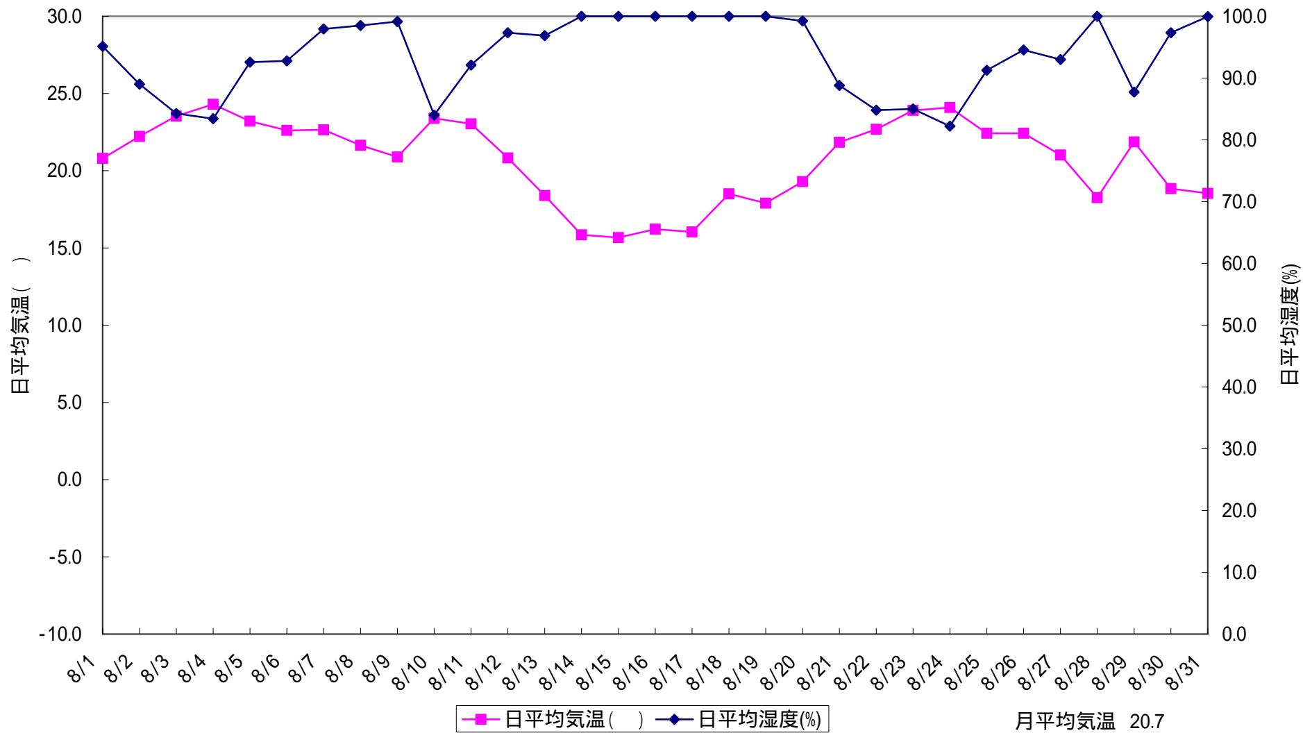
図 日平均気温と日平均湿度(群馬県川場村ヒロイド 2003/8)
