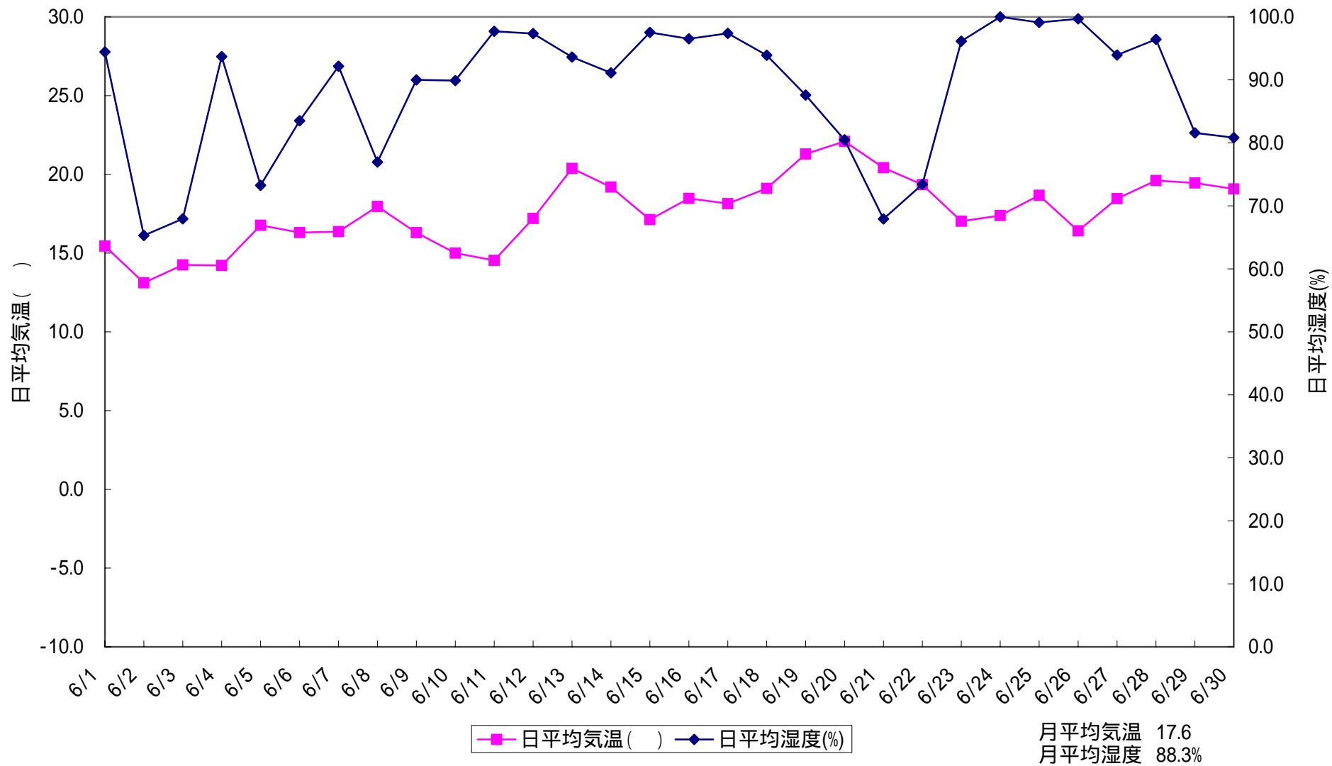
図 日平均気温と日平均湿度(群馬県川場村ヒロイド 2003/6)
