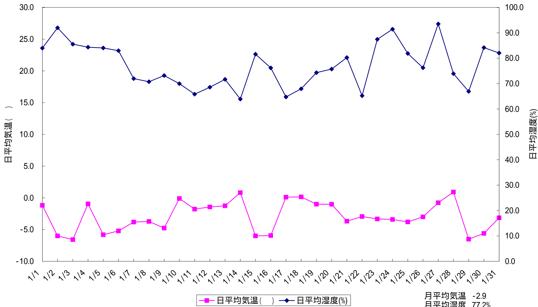
図 日平均気温と日平均湿度(群馬県川場村ヒロイド 2003/1)
