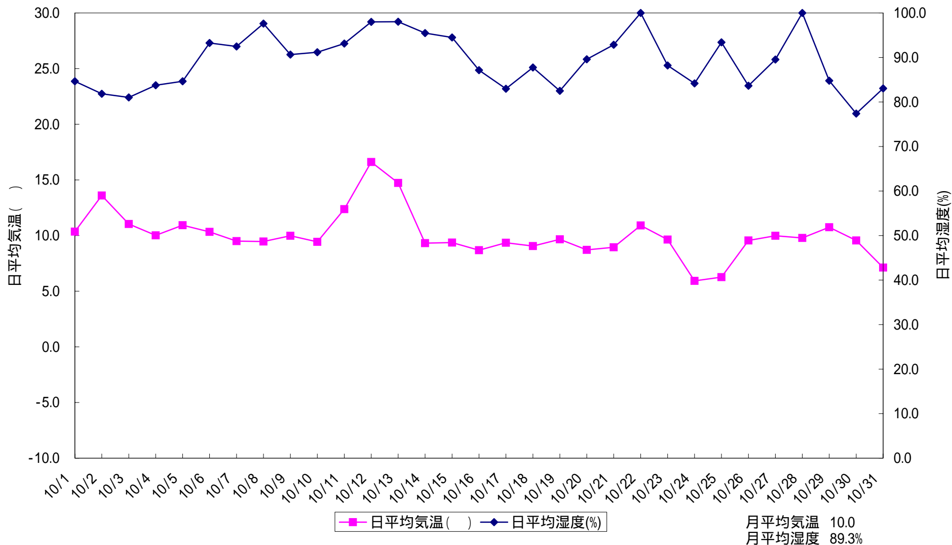
図 日平均気温と日平均湿度(群馬県川場村ヒロイド 2003/10)
