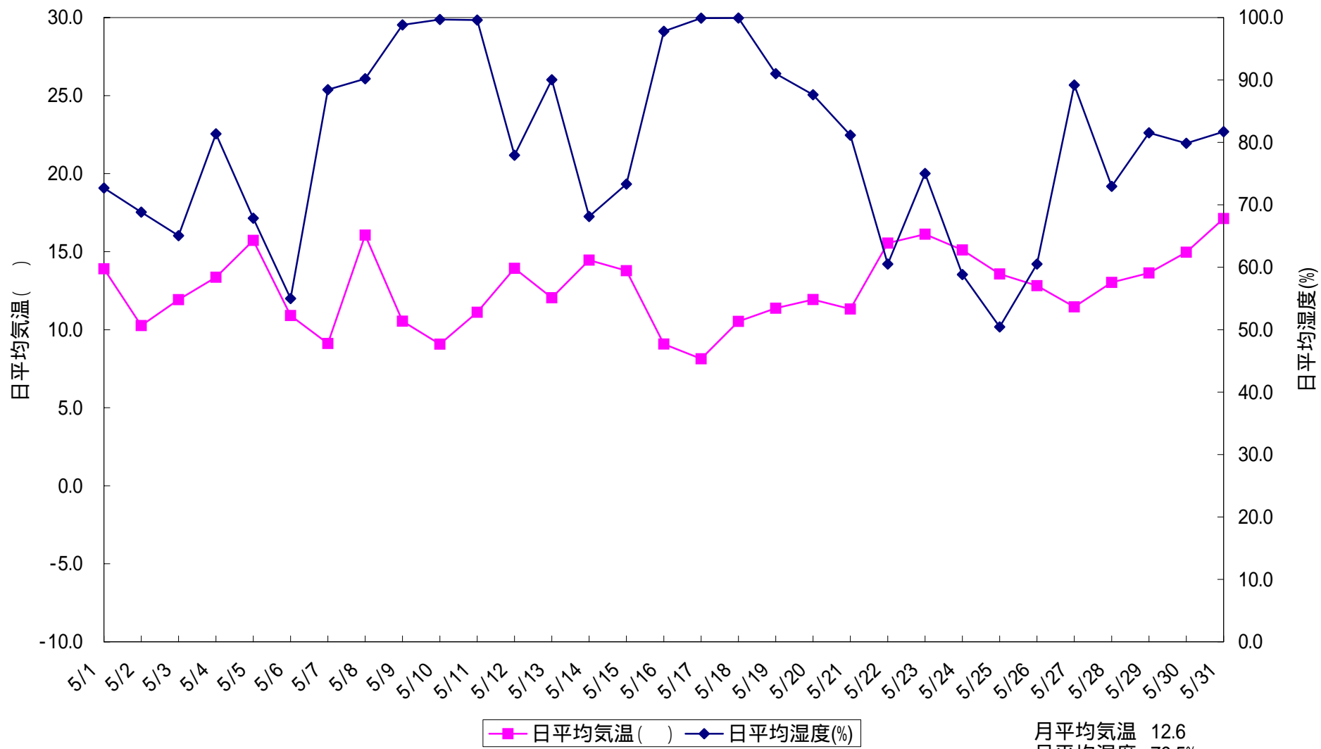
図 日平均気温と日平均湿度(群馬県川場村 2002/5)
