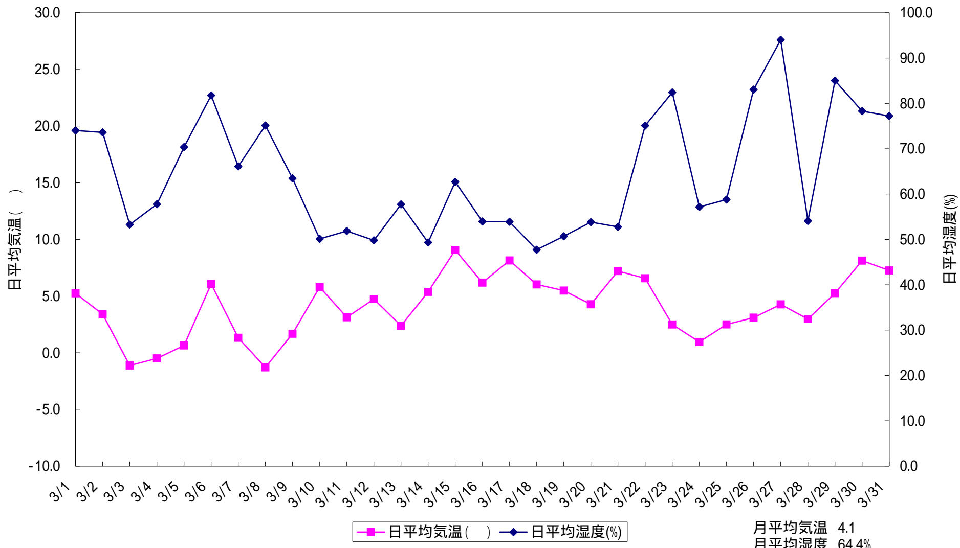
図 日平均気温と日平均湿度(群馬県川場村 2002/3)
