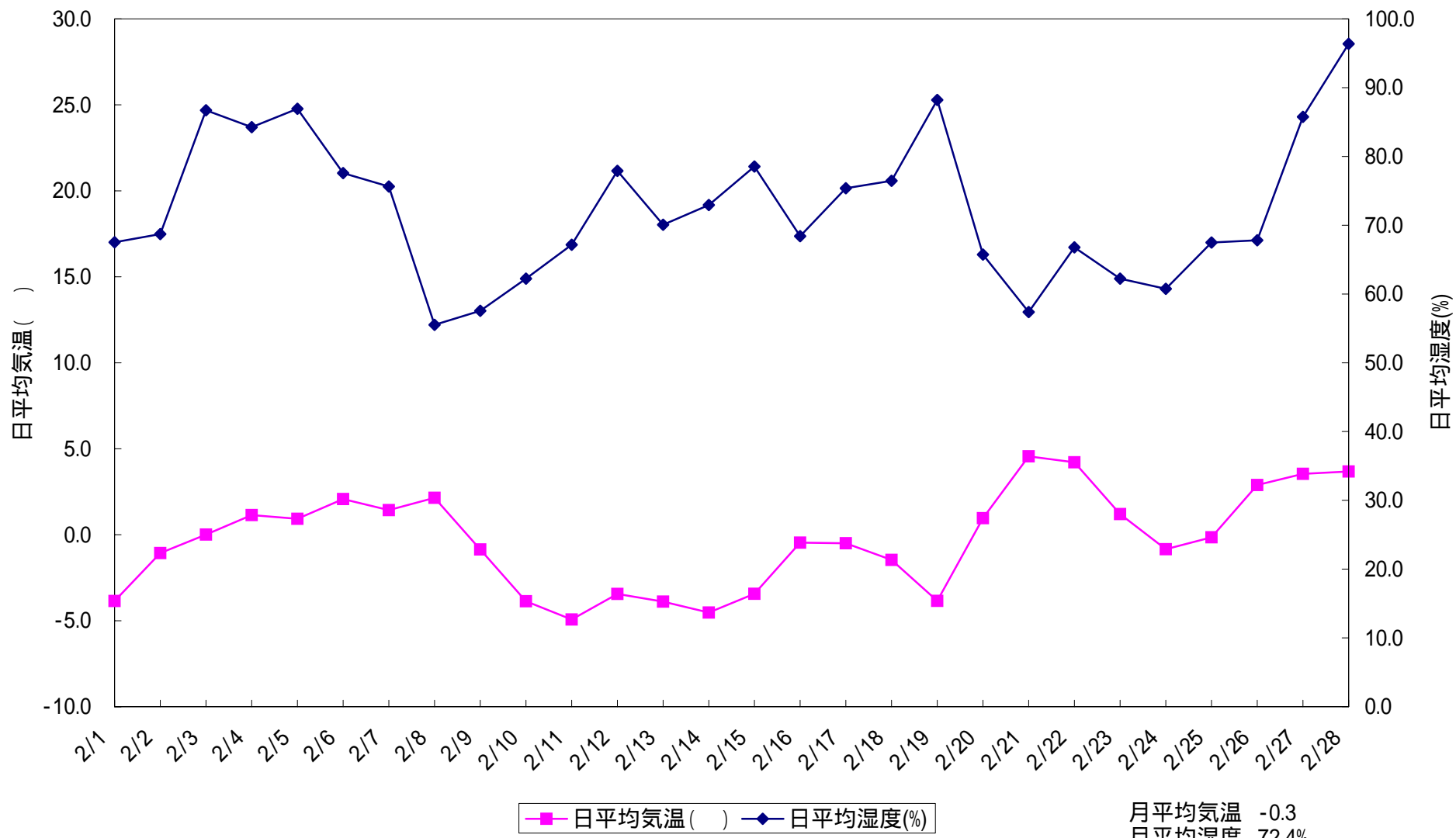
図 日平均気温と日平均湿度(群馬県川場村 2002/2)
