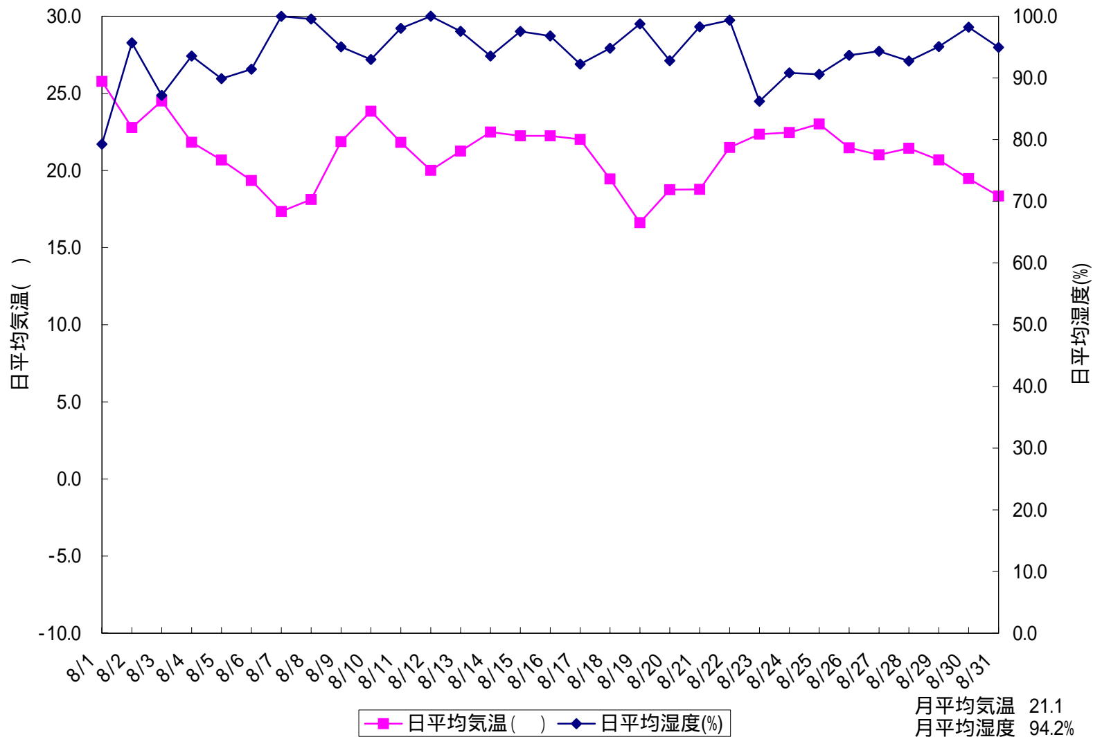
図 日平均気温と日平均湿度(群馬県川場村ヒロイド 2001/08/01 ~ 2001/08/31)
