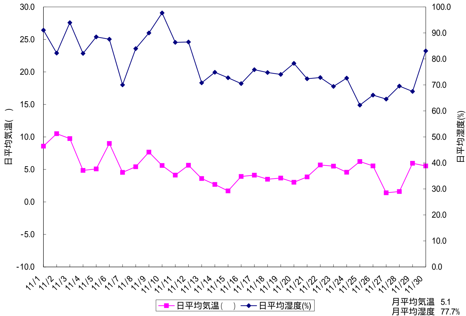
図 日平均気温と日平均湿度(群馬県川場村ヒロイド 2001/11/01 ~ 2001/11/30)
