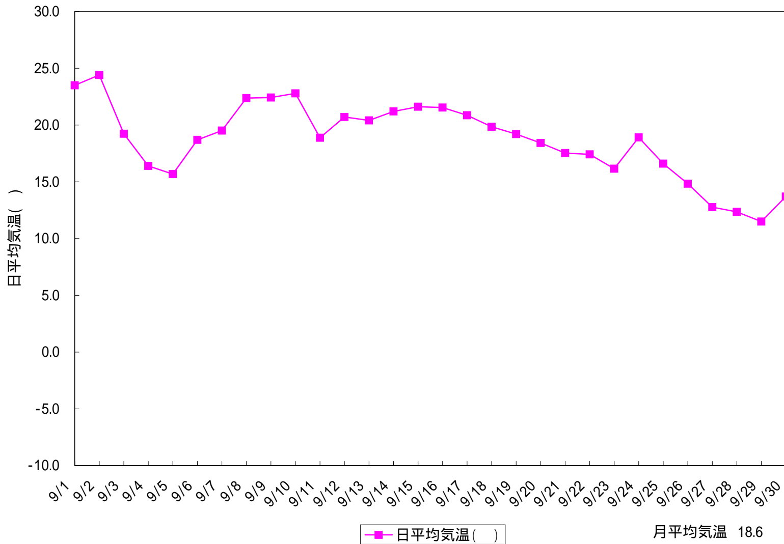
図 日平均気温(群馬県川場村ヒロイド 2000/09/01 ~ 2000/09/30)
