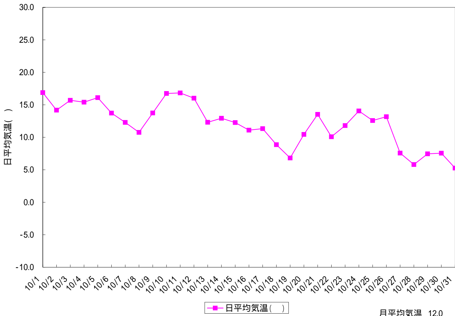
図 日平均気温(群馬県川場村ヒロイド 2000/10/01 ~ 2000/10/31)
